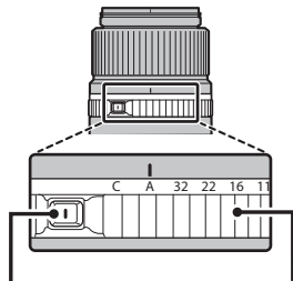
Przycisk zwolnienia blokady pierścienia przysłony
