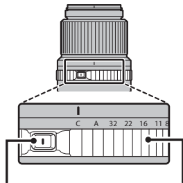
Przycisk zwolnienia blokady pierścienia przysłony Pierścień przysłony
