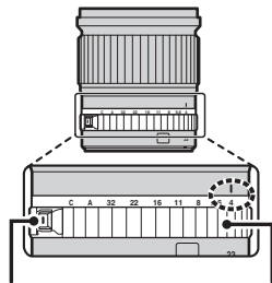
Himmenninrenkaan lukituksen vapautus
